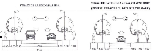
PROFIE TRANSVERSALE CARACTERISTICE PENTRU DRUMURILE PROPUSE PE TRASEE NOI SI PENTRU REABILITARE cote minime
